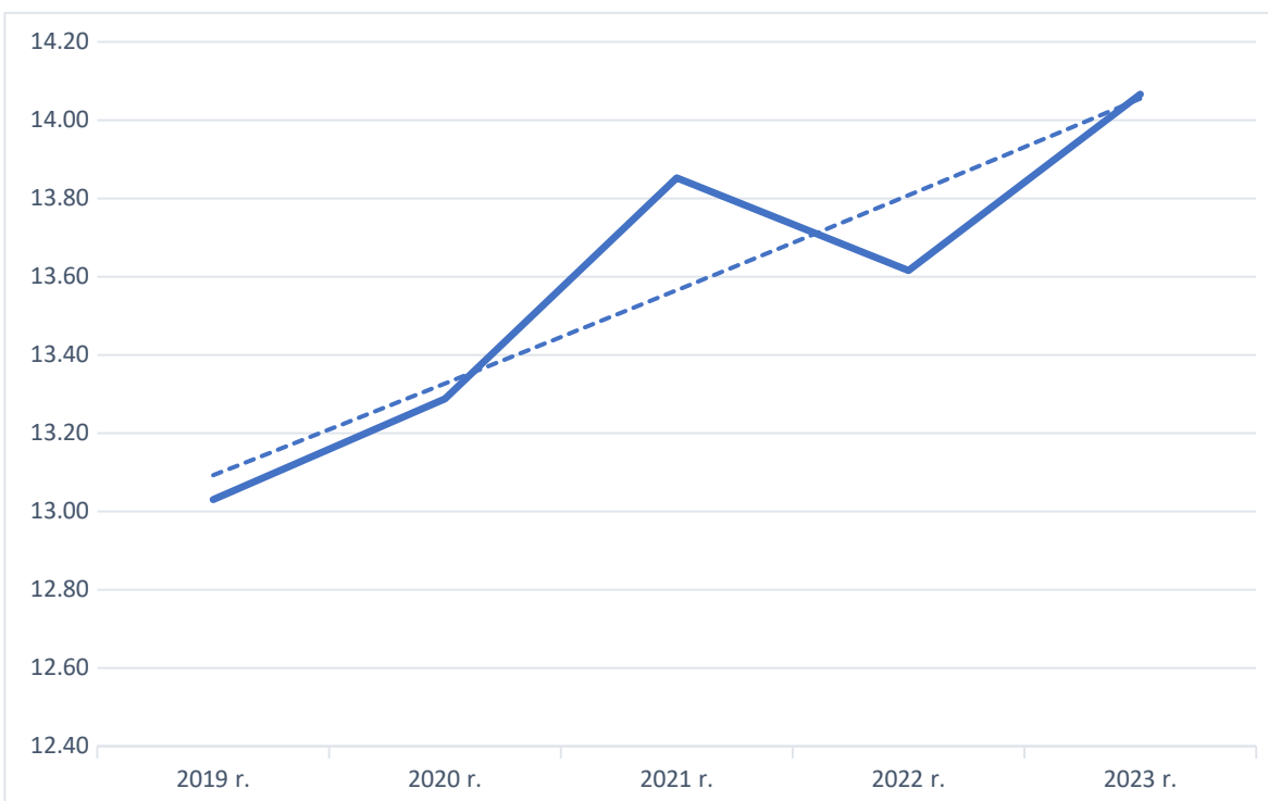
Wykres 6. Szacowane łączne zużycie energii elektrycznej [GWh] w gminie Starożreby
