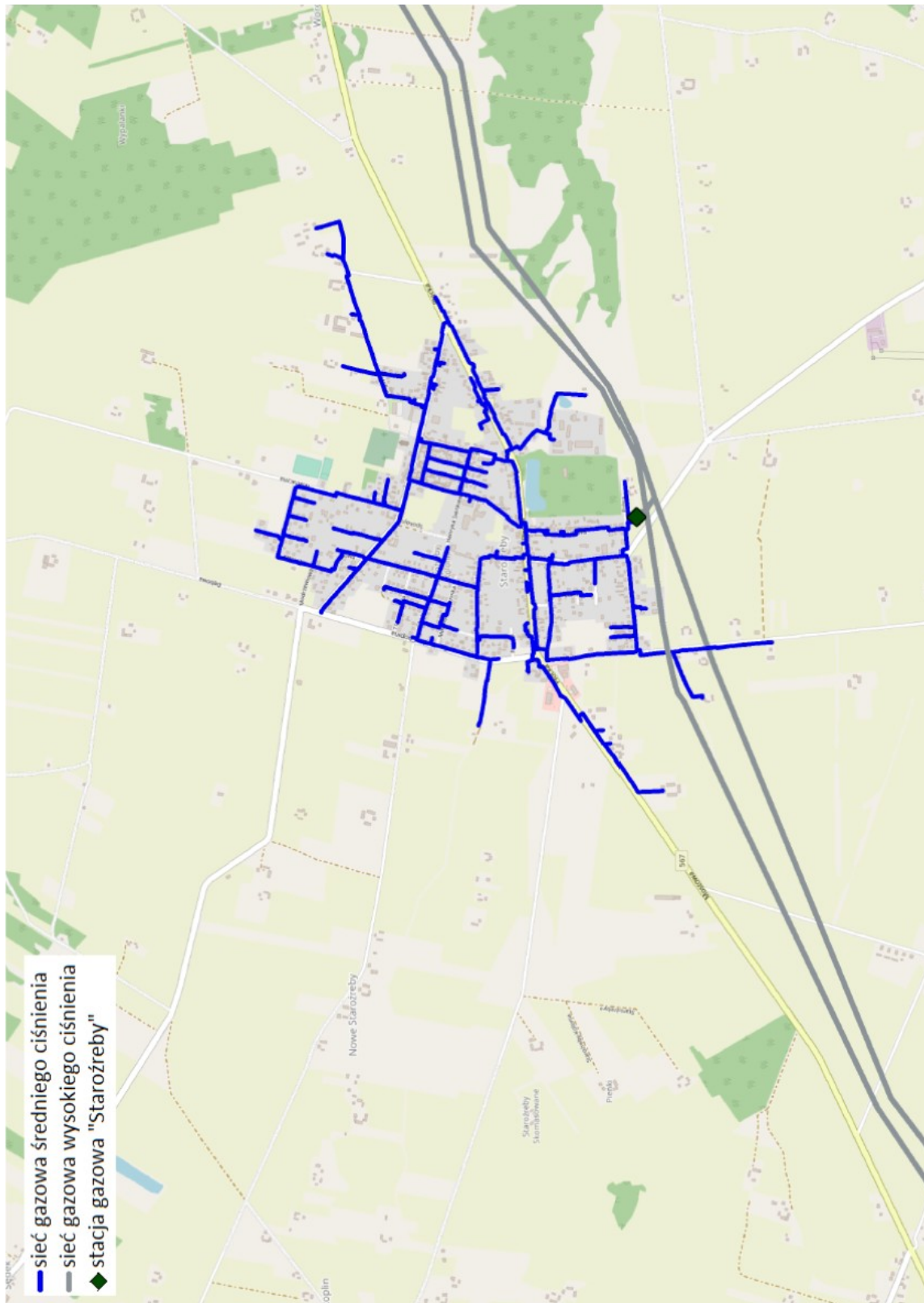
Rysunek 4. Infrastruktura Polskiej Spółki Gazownictwa Sp. z o.o. na terenie gminy Starożreby
